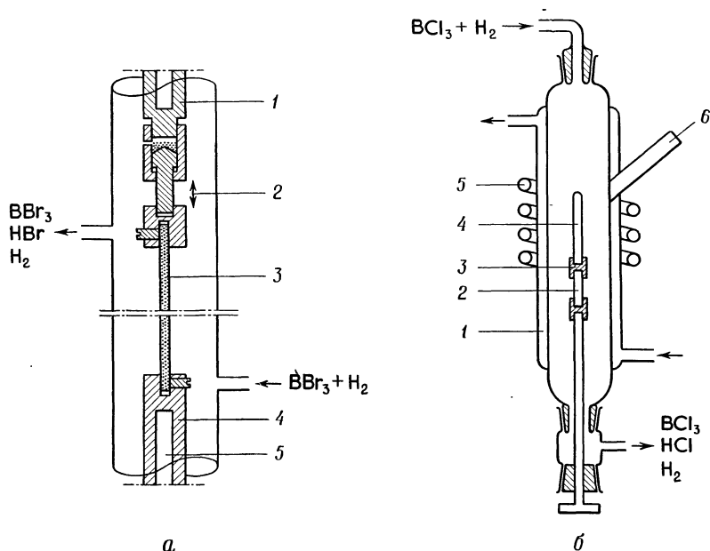
Рис. 15. Аппарат, применяющийся для восстановления \text{VBr}_3 водородом на подложке из бора.
