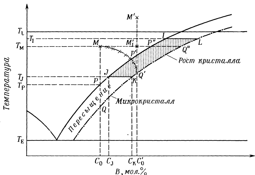
Рис. 26. Фазовые соотношения в двойных системах, иллюстрирующие различия между двумя методами роста из раствора в расплаве: изотермическим испарением флюса и медленным охлаждением.
