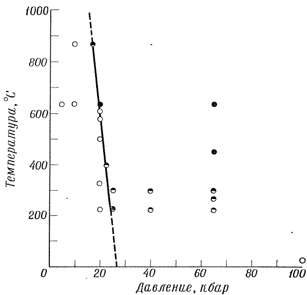
Рис. 13б. Фазовая диаграмма давление—температура для \text{RbNiF}_3 [87]. \circ — гексагональная фаза; \bullet — кубическая фаза.
