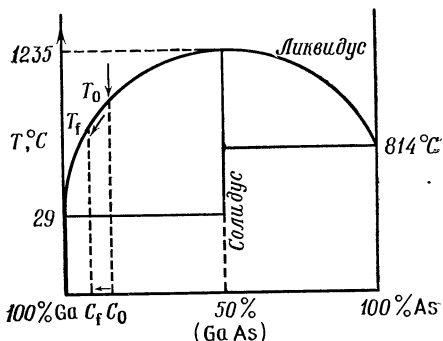
Рис. 17. Жидкостная эпитаксия; фазовая диаграмма для GaAs.
