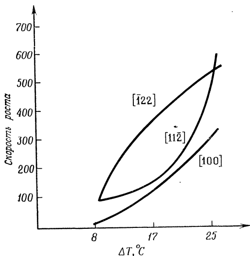
Рис. 38. Скорость роста V (мкм·сут -1 ·грань -1 ) \text{Al}_2\text{O}_3 в 4 М растворе \text{Rb}_2\text{CO}_3 ; степень заполнения 85%; T=442^\circ\text{C} [87].
