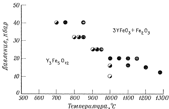
Рис. 16. Фазовая диаграмма давление—температура для Y_3Fe_5O_{12} [110].
