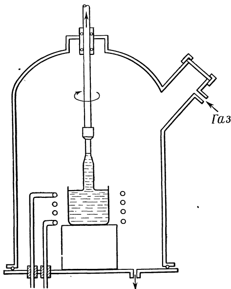
Рис. 2. Аппарат Чохральского [1].
