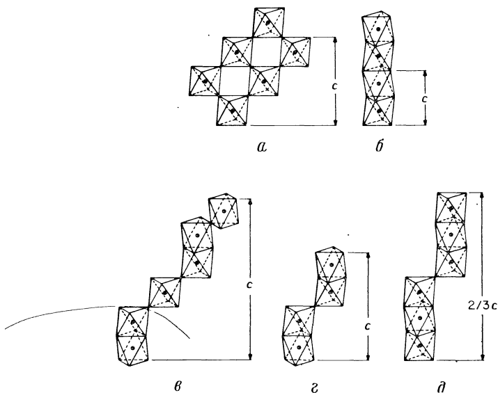
Рис. 4. Стабильные структуры, промежуточные между кубическим перовскитом (а) и 2H -структурой CsNiCl_3 (б): 6H -структура BaTiO_3 (в), 4H -структура SrMnO_3 (г), 9R -структура BaRuO_3 (д).
