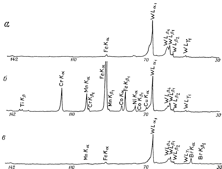
Рис. 7. Рентгеноспектральный анализ (вольфрамовая трубка) чистого бора, полученного восстановлением \text{BBr}_3 водородом при 1300^\circ\text{C} на танталовой нити (а), промышленного образца бора, применяющегося для синтеза \text{BBr}_3 (б), и чистого бора, полученного восстановлением \text{BBr}_3 водородом при 750^\circ\text{C} на внутренней стенке кварцевой трубки (в).
