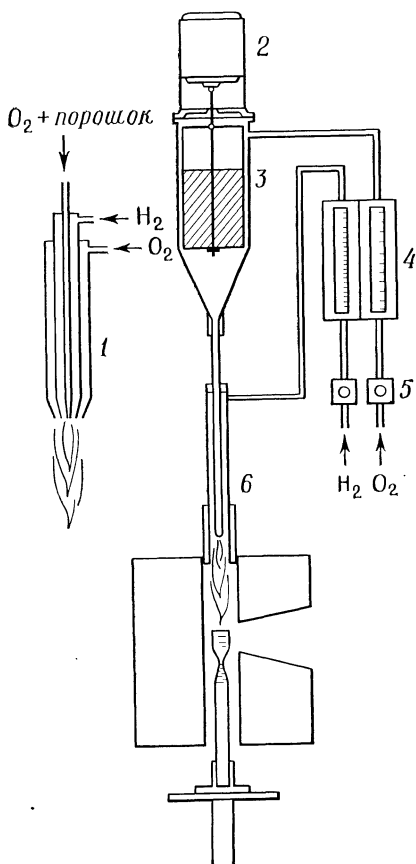
Рис. 8. Аппарат Вернейля [1].
