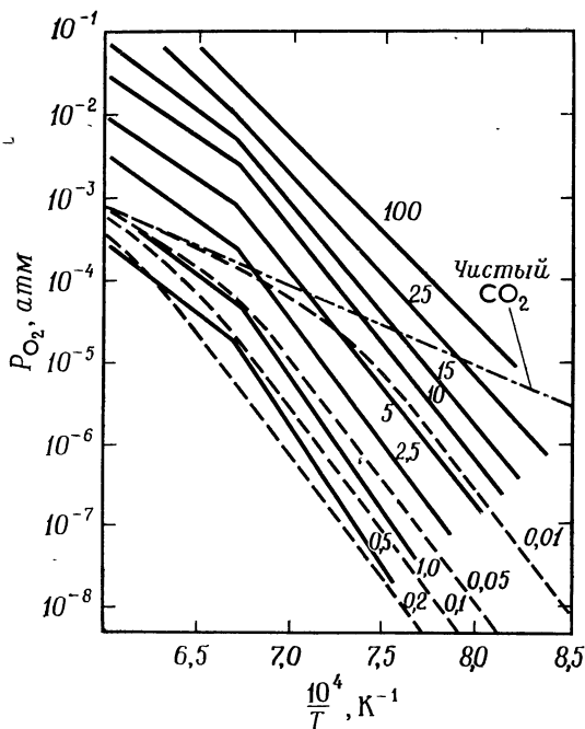
Рис. 6. Диаграмма с линиями равного состава для \text{Co}_{0.165}\text{Fe}_{0.835}^{2+}\text{Fe}_2\text{O}_4 .
