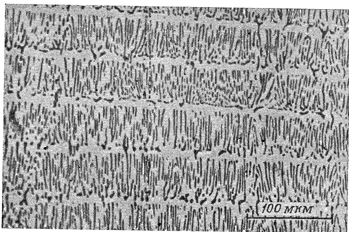
Рис. 20. Продольный разрез образца композитного материала \text{MnSb—Sb} стержневого типа, проявляющего полосчатость ( \times 275 ).
