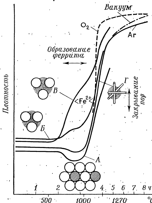
Рис. 14. Схематическое изображение кривых плотности Mn, Zn-ферритов для различных размеров, формы и упаковки частиц и разных атмосфер. Для одной постоянной атмосферы содержание \text{Fe}^{2+} увеличивается по мере возрастания температуры закрывания пор [22].
