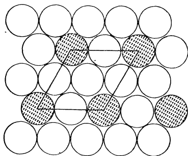
Рис. 2. Плотнупакованный слой AX_3 , в котором видны положения катионов А (затемненные кружки) и анионов Х (светлые кружки).
