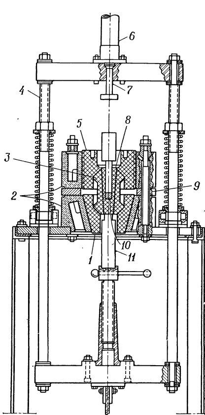
Рис. 1. Схема пресса для горячего прессования [30].
