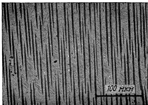
Рис. 5. Сечение, параллельное направлению роста (снизу вверх). эвтектики MnSb—Sb, характеризующейся стержневидными кристаллитами.
