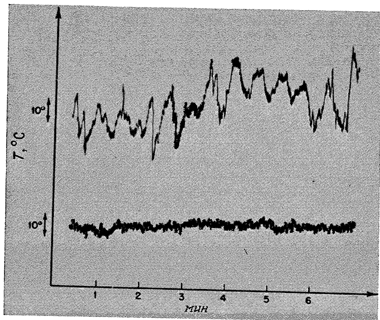
Рис. 15. Колебания температуры вблизи 200 °C в горячей зоне зеркальной радиационной печи. Вверху : источник с графитовой вольтовой дугой. Внизу : источник — ксеноновая дуговая лампа.
