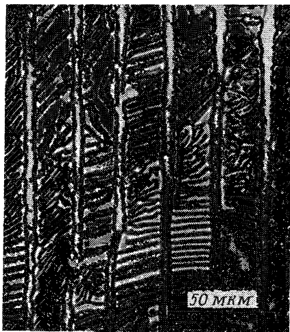
Рис. 22. Продольный разрез комбинированного композитного материала Co-(Co-Co_2Si) ; \times 500 .
