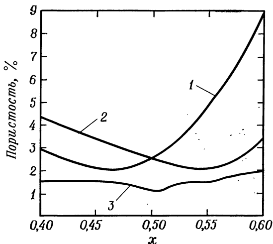
Рис. 20. Пористость никелевых ферритов, спекавшихся при 1350^\circ\text{C} в течение 24 ч в кислороде (1), смеси азот+1% кислорода (2) и азоте (3) в зависимости от параметра состава x для системы (1-x)\text{NiO} + x\text{Fe}_2\text{O}_3 . [71].
