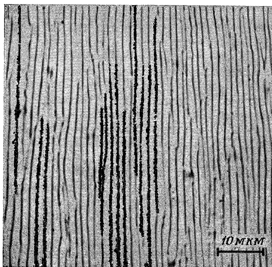
Рис. 9. Эвтектическая пленка \text{Cd-Zn} , выращенная в проволочной петле дольный разрез снизу вверх; \times 1480 ).
