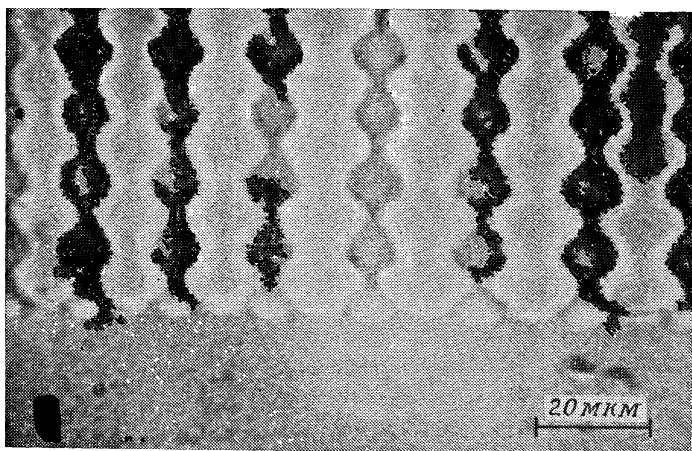
Рис. 19. Модуляция ламелл эвтектики \text{AgCl—CuCl} ( \times 900 ) [54].
