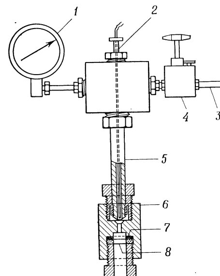
Рис. 5. Реактор высокого давления Келли и сотр. [88].
