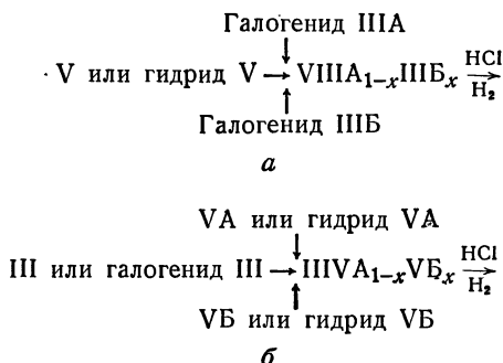
Рис. 20. Реакции, протекающие при выращивании эпитаксиальных пленок тройных твердых растворов в открытом реакторе.
