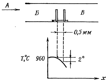
Рис. 13. Система для эпитаксиального осаждения методом близкого переноса, держатель образцов и температурный профиль.
