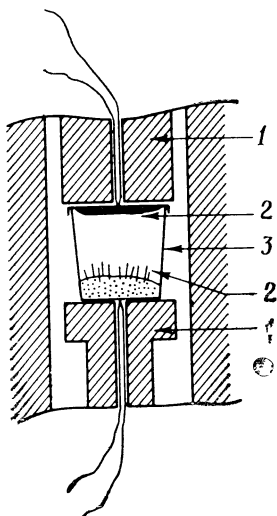
Рис. 10. Выращивание кристаллов WO_3 [4].
