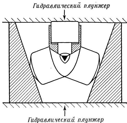
Рис. 28. Схематический чертеж упрощенного тетраэдрического аппарата [154].
