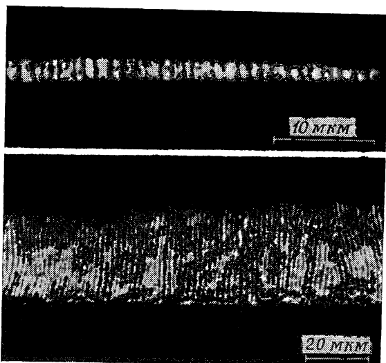
Рис. 10. Эвтектическая пленка \text{Cd-Zn} , выращенная в проволочной петле перечное сечение; \times 2400 ).
