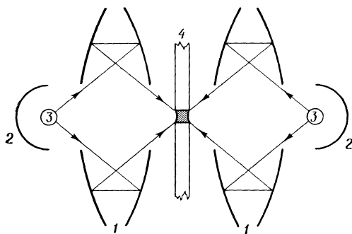
Рис. 18. Оптическая система с двумя зеркальными радиационными нагревателями [17].
