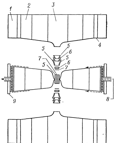
Рис. 25. Аппарат типа «белт» для работы при высоких температурах и давлениях; чертеж со «смещенной» детализировкой [148].
