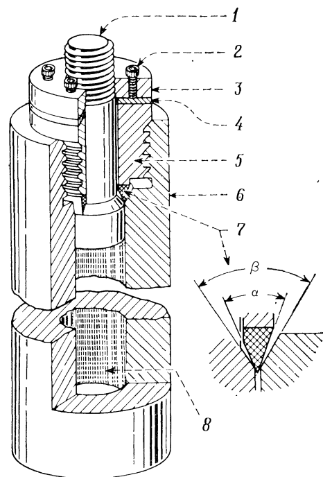
Рис. 35. Автоклав Бриджмена [23].
