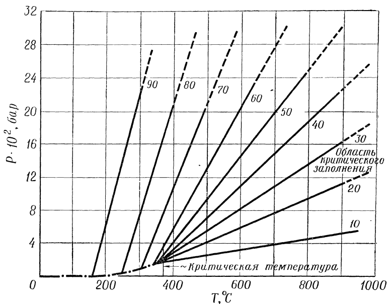
Рис. 32. Кривые давление—температура для воды при постоянном объеме [80]. Цифрами на кривых указана степень заполнения, %; — — кривая сосуществования \text{H}_2\text{O} (газ) + \text{H}_2\text{O} (жидк.).
