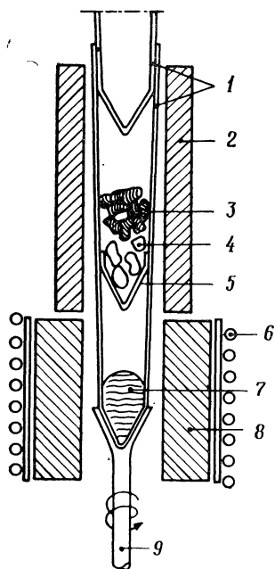
Рис. 5. Синтез GaP и выращивание кристаллов в разборной ампуле из пиролитического нитрида бора [15].
