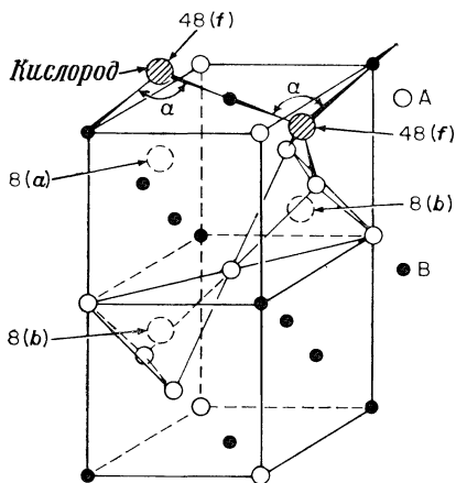
Рис. 8а. Катионная подрешетка для одной четверти элементарной ячейки кубической структуры пироксера. Показаны также два из 48 (f) анионов [58].
