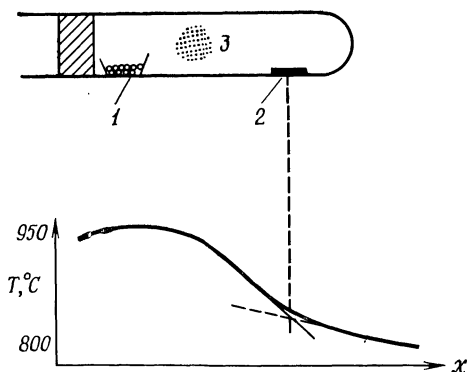
Рис. 7. Транспорт GaP в запаянной трубке при помощи йода.
