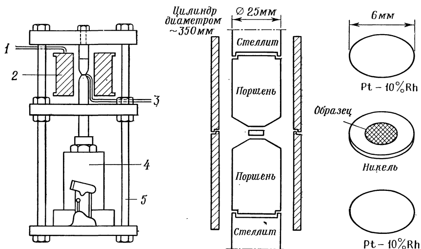
Рис. 19. Схематическое изображение аппарата с плоскопараллельными наковальными [135].
