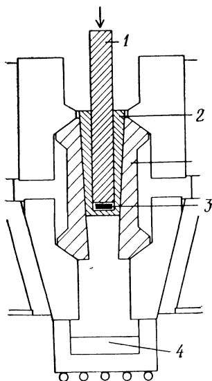
Рис. 2. Экспериментальная установка для исследования закалки карбидов.
