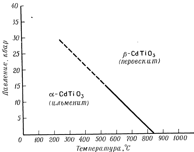
Рис. 17. Фазовая диаграмма давление—температура для CdTiO_3 [115].
