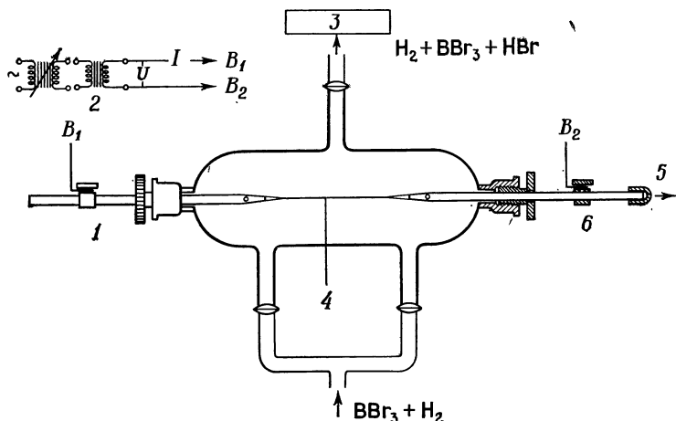
Рис. 12. Ампула с горячей нитью для восстановления \text{VBBr}_3 водородом при высокой температуре.
