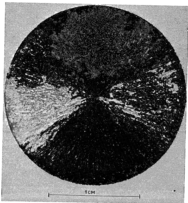
Рис. 25. Радиально ориентированная кристаллизация стержней \text{Sr}_7\text{C}_3 в матрице Fe (поперечный разрез; \times 5,7 ) [61].
