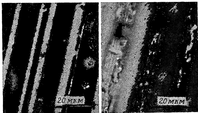
Рис. 14. Поверхность композитного материала \text{SnSe}-\text{SnSe}_2 после отжига со смесью \text{Sn}+\text{SnSe} [44].
