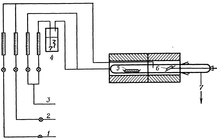
Рис. 9. Процесс \text{Ga}-\text{AsCl}_3 .
