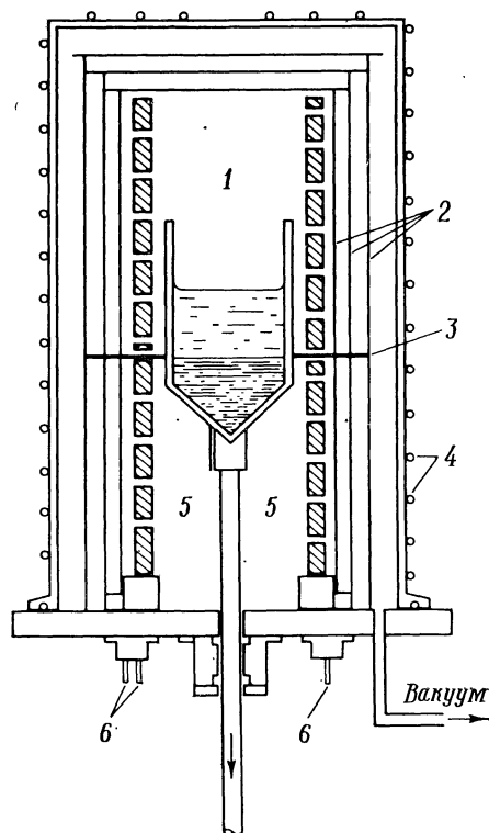
Рис. 3. Аппарат Бриджмена—Стокбаргера [1].
