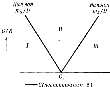
Рис. 18. Зависимость G/R от концентрации в области регулярного роста композитного материала.
