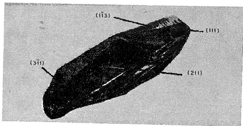
Рис. 39. Кристалл рубина, выращенный в гидротермальных условиях [87].
