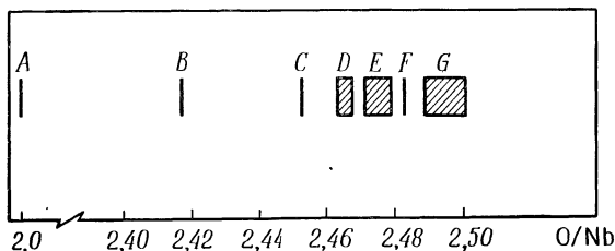
Рис. 2. Термодинамически устойчивые фазы окиси ниобия в пределах от \text{NbO}_2 до \text{NbO}_{2,5} при 1300^\circ\text{C} [77].
