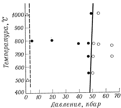
Рис. 13а. Фазовая диаграмма давление—температура для \text{CsNiF}_3 [86]. \Delta — слой 2; \bullet — слой 9; \circ — слой 6.
