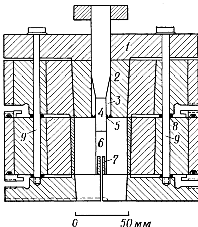
Рис. 24. Двухступенчатая поршневая система [144].
