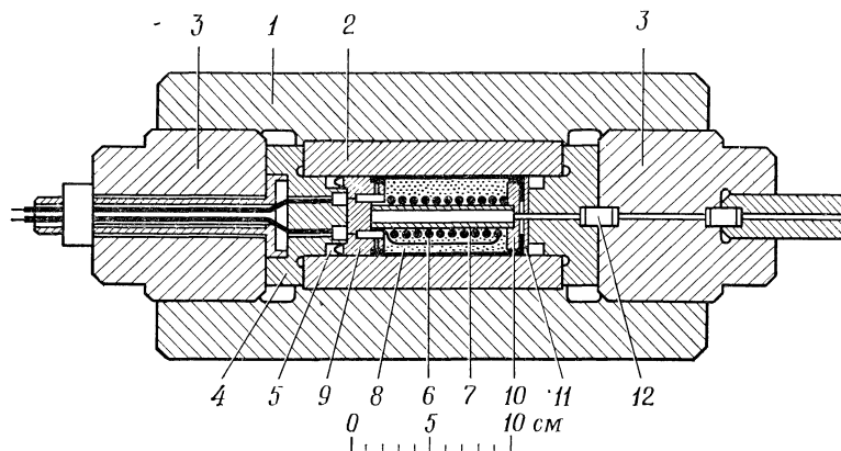
Рис. 3. Поперечный разрез газового автоклава, сконструированного Вильгельми [9].
