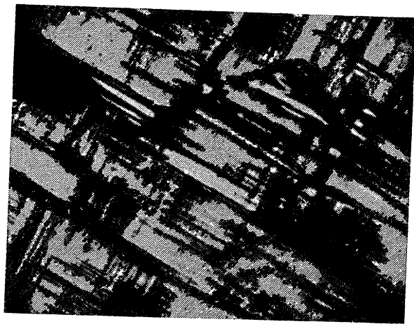
Рис. 43. Двойниковые структуры в кристалле \text{Ba}_2\text{NaNb}_5\text{O}_{15} ( \times 10 ) [118].
