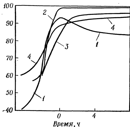
Рис. 12. Кривые уплотнения для ферритов, полученных соосаждением из разных растворов [37]. На оси ординат указана степень достижения теоретической плотности (%).
