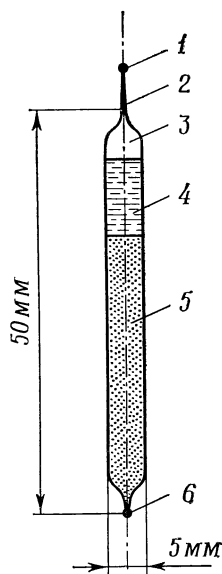
Рис. 1. Запаянная трубка из золота для гидрофторотермального синтеза [15].
