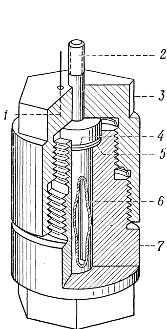
Рис. 12. Бомба Моури для гидротермальных реакций [49].
