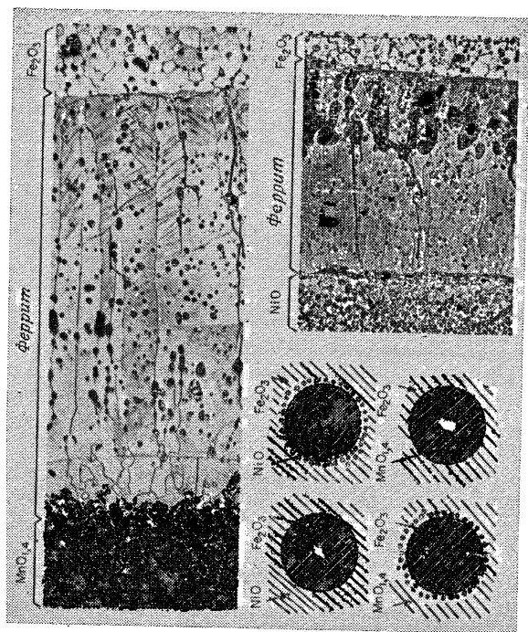
Рис. 10. Диффундирующие пары окисей в процессе образования марганцевого и никелевого ферритов [22].
