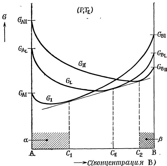
Рис. 1. Эвтектическое равновесие.
