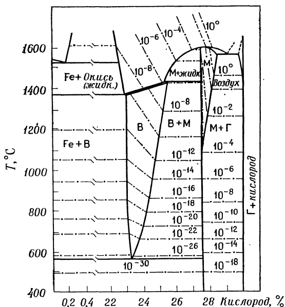
Рис. 4. Система Fe—O— [3].
