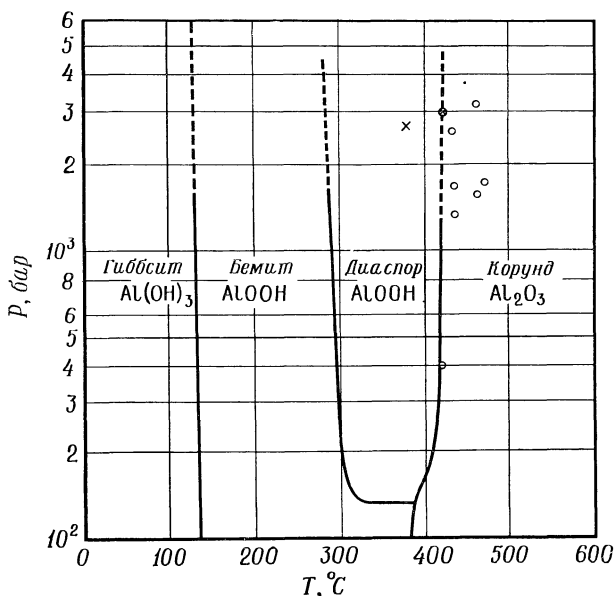
Рис. 37. Система \text{Al}_2\text{O}_3\text{--H}_2\text{O} [23].
