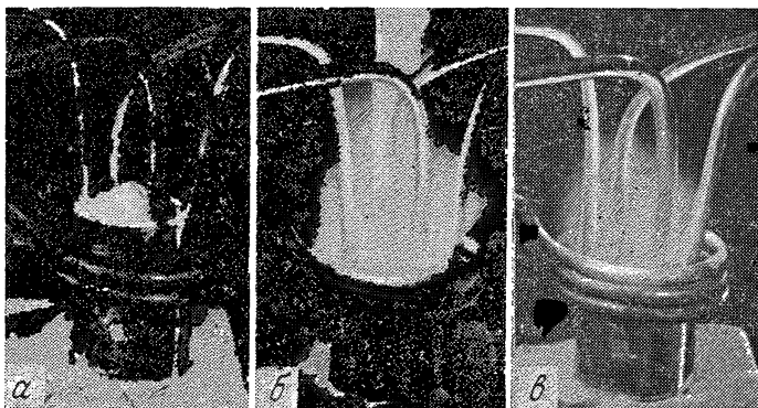
Рис. 20. Бестигельное плавление [19].
