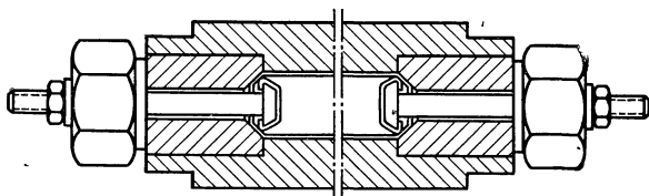
Рис. 15. Самоуплотняющийся автоклав [60].
